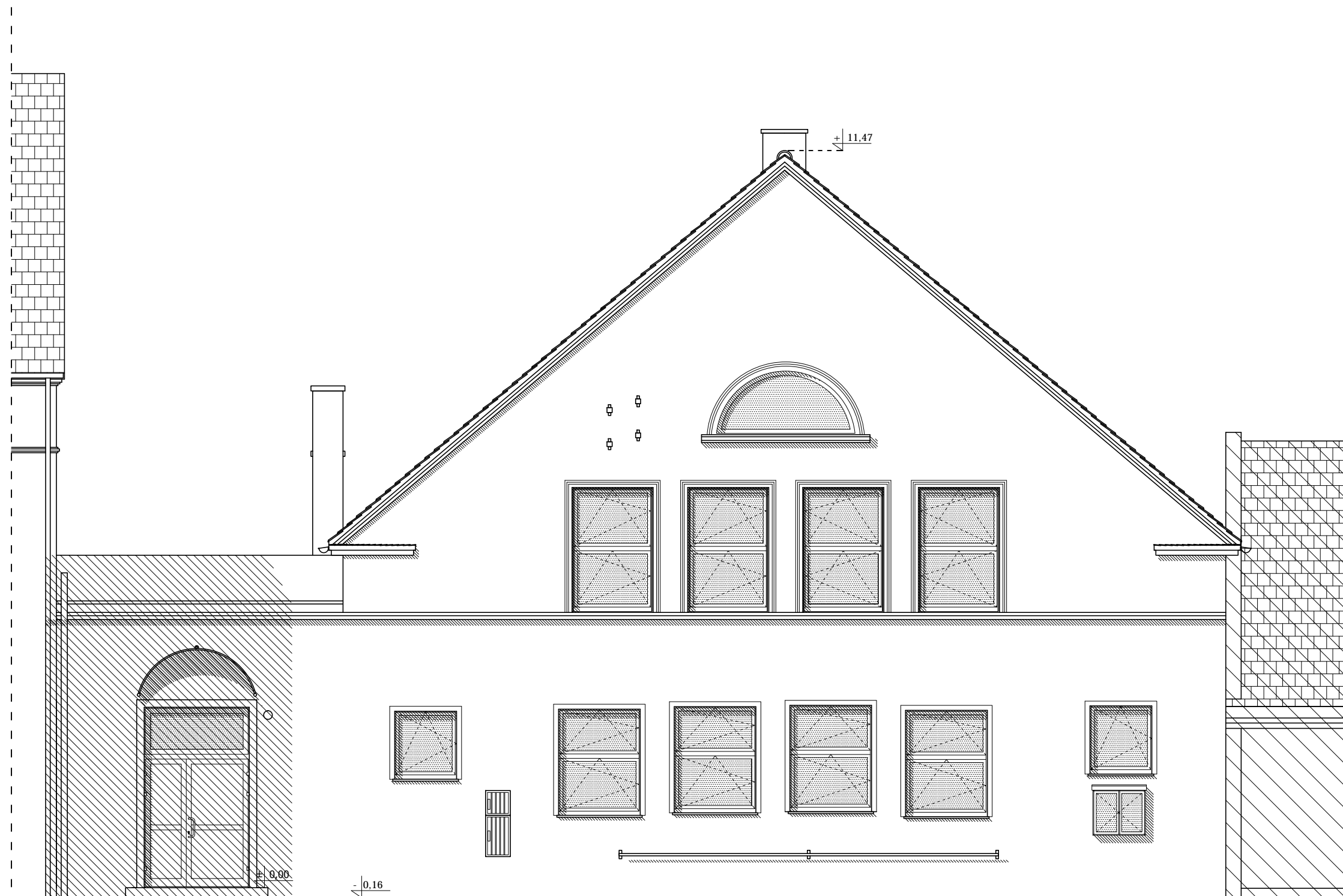
ELEWACJA POŁUDNIOWA
