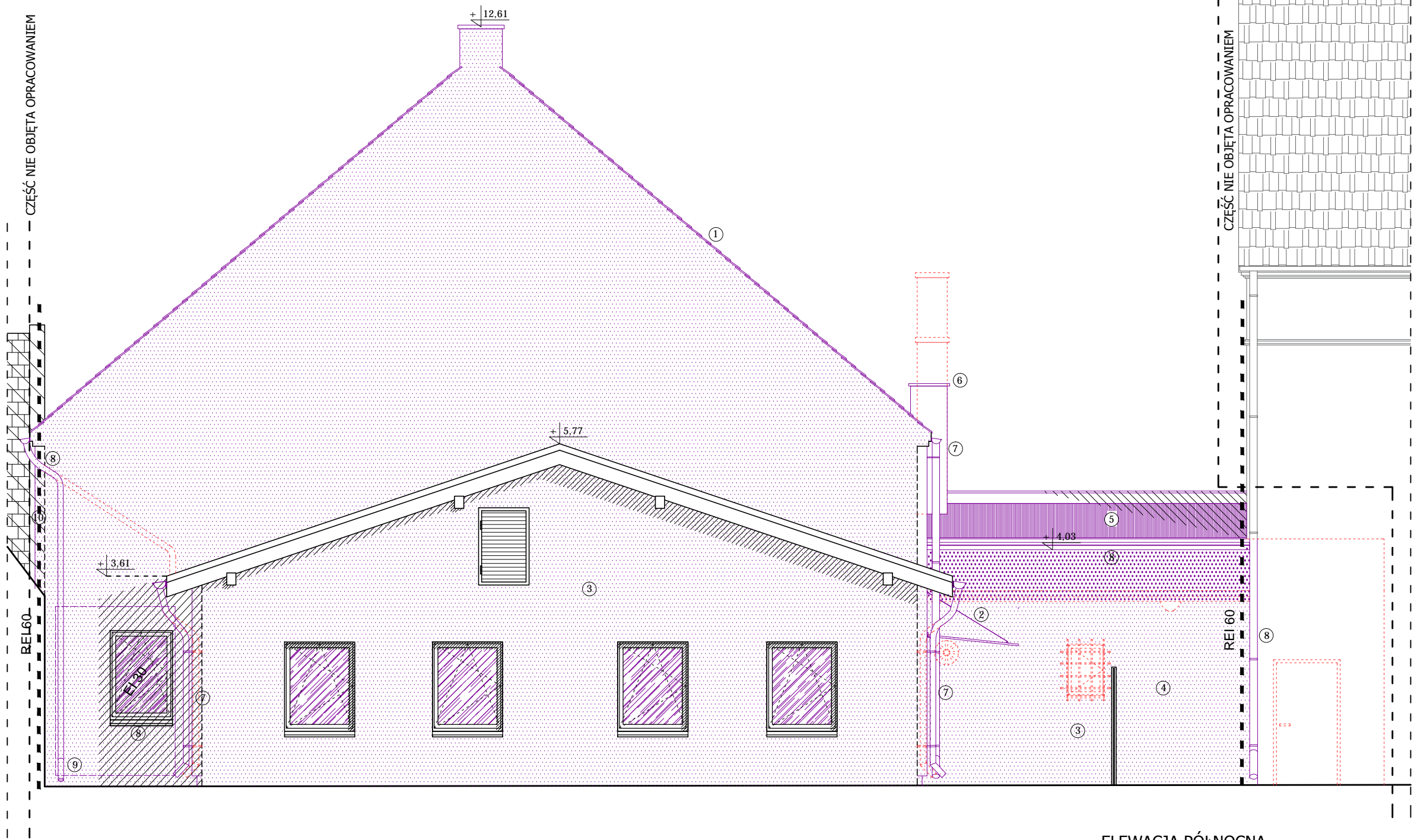
ELEWACJA PÓŁNOCNA
